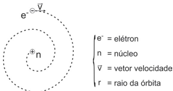
Figura 16: Colapso do elétron no núcleo
