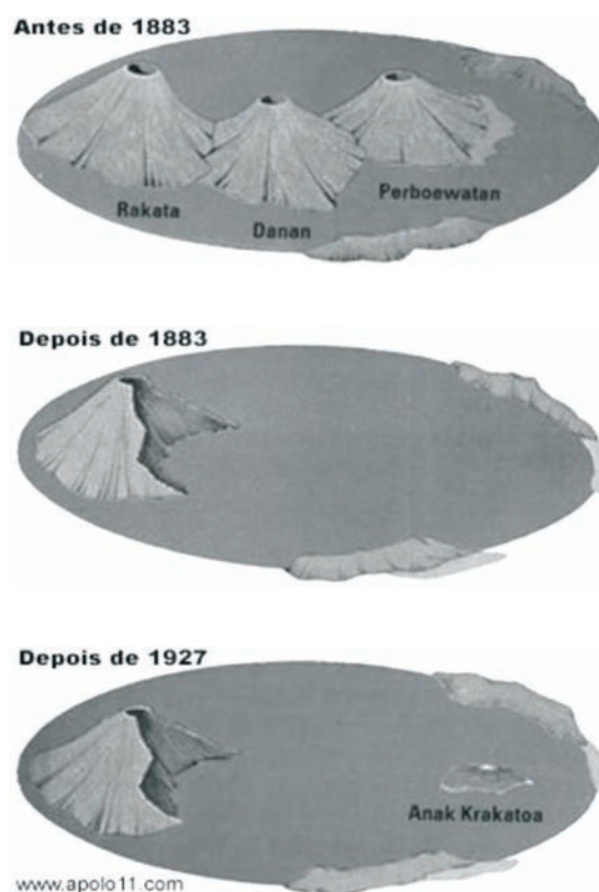
Figura 12: Vulcões.
