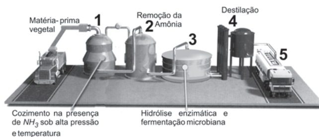
Figura 26: Decomposição da celulose com amônia.
